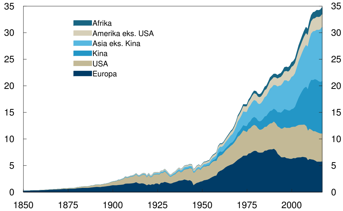
Figur 11 Utslipp øker i fremvoksende økonomier. CO 2 -utslipp. Gigatonn
